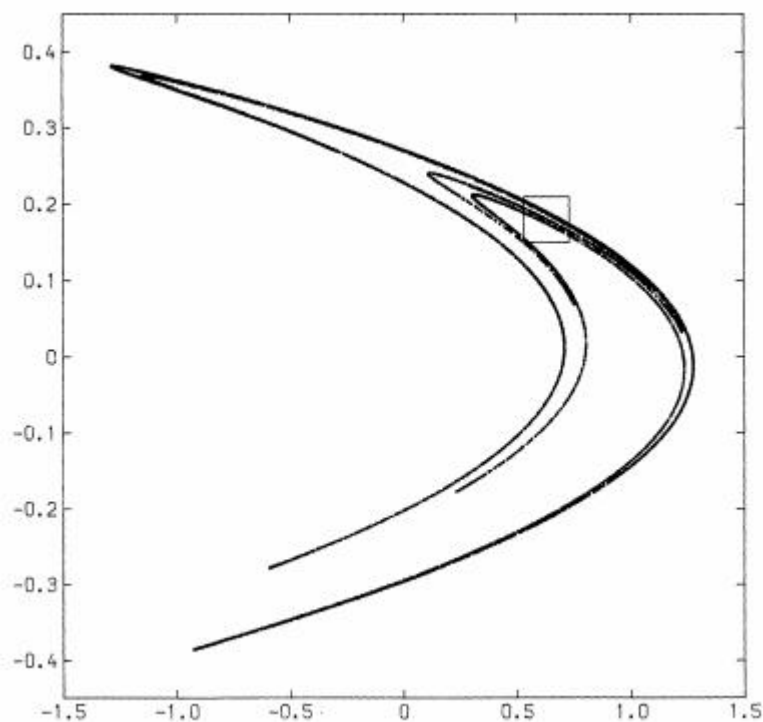
图 3。与图 2 相同，但是从 x_0=0.63135448, y_0=0.189406341 开始。
