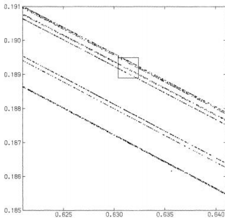
图 5 所示。图 4 的平方区域放大: n=10^6
