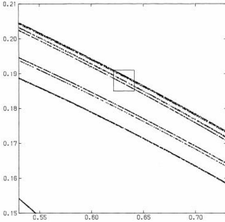
图 4 所示。图 3 的平方区域的放大。计算的点数增加到 n=10^5 。
